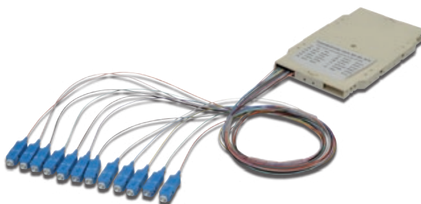
Spleißkassette mit 12 SC-Pigtails Splice Cassette with 12 SC Pigtails
